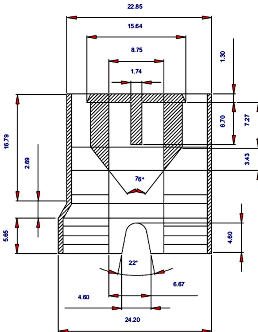
Base para Relé Auxiliar Automotivo 5 terminais Faston 6.3mm UC3003/4
